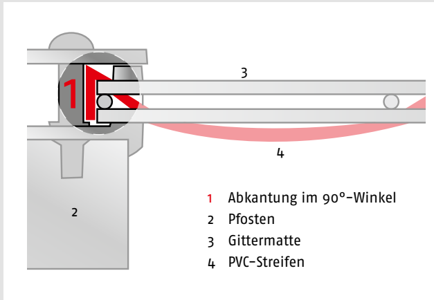
Abkantung Draufsicht
